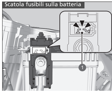
1 Bruciato
