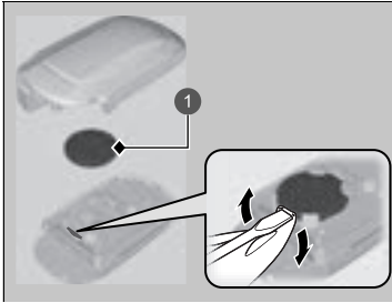
1 Batteria
