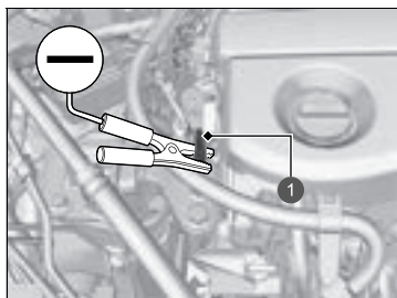
1 Bullone prigioniero
