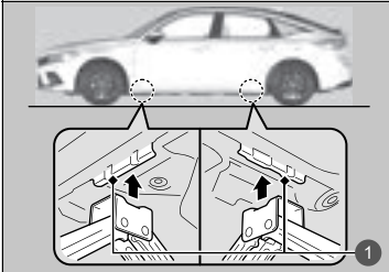
1 Punti di sollevamento
